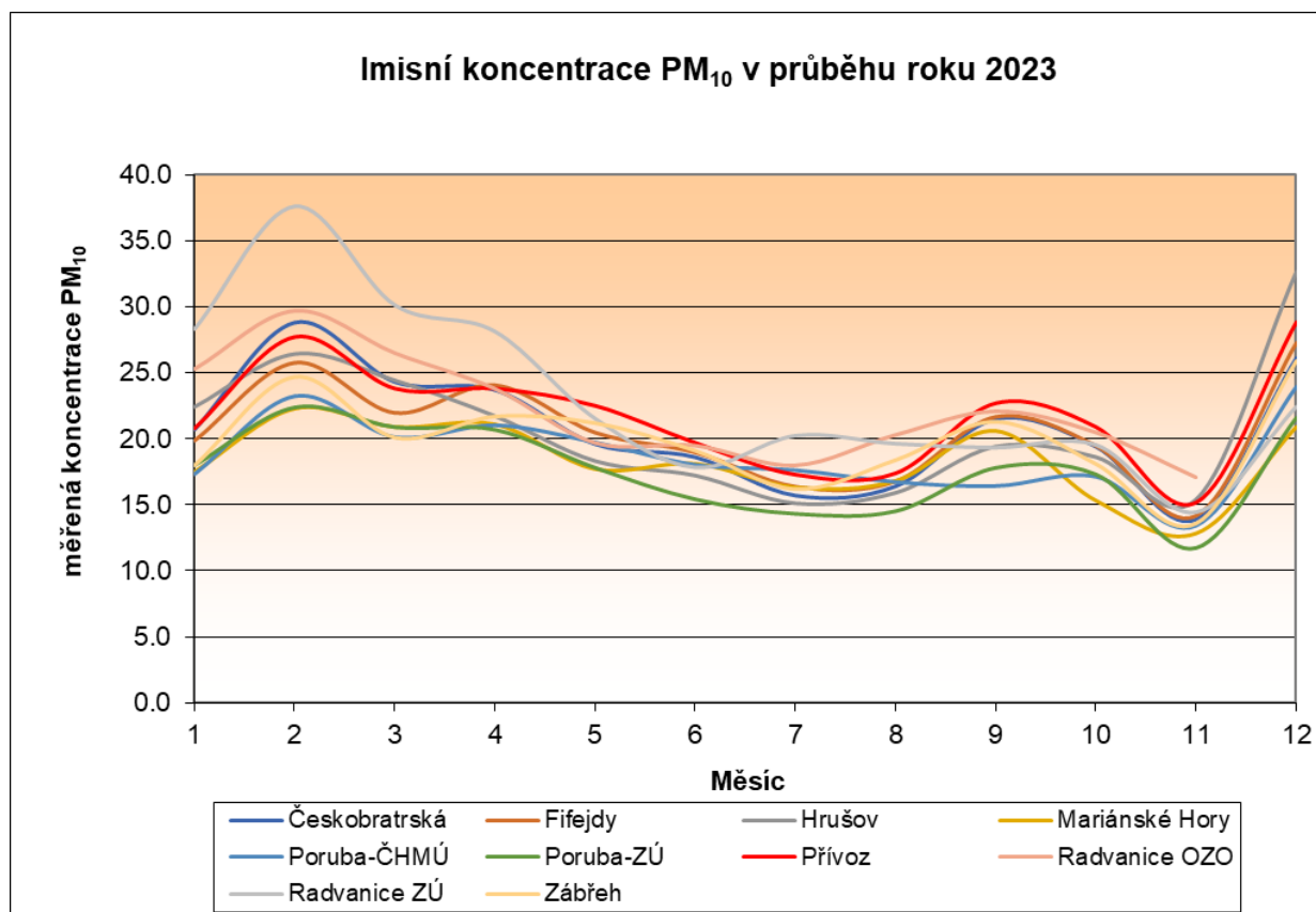
Obrázek 23 Roční chod imisních koncentrací PM 10 v roce 2023 [µg/m 3 ] Okres Ostrava – město
