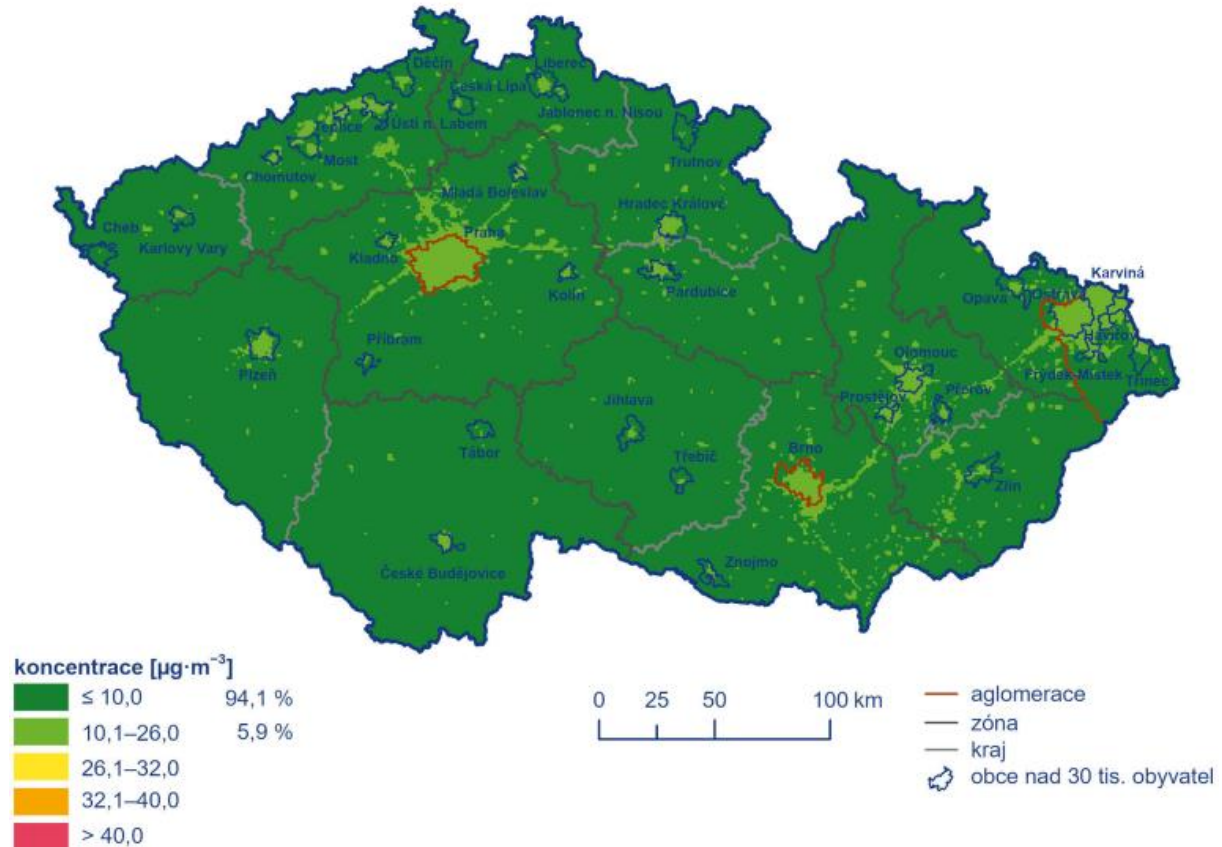
Obrázek 35 - Pole roční průměrné koncentrace NO 2 v ČR v roce 2023
