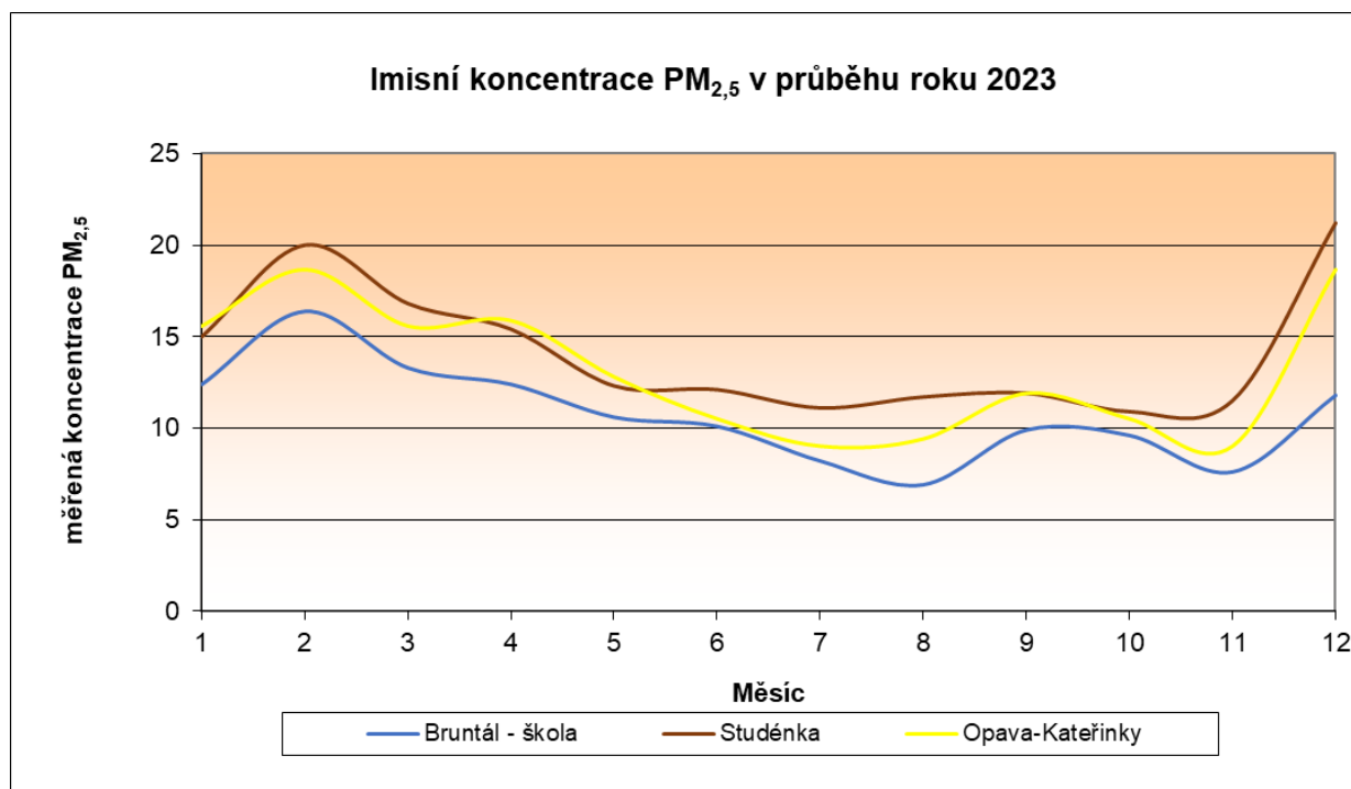
Obrázek 28 Roční chod imisních koncentrací PM 2,5 v roce 2023 [µg/m 3 ] Okresy Bruntál, Nový Jičín, Opava
