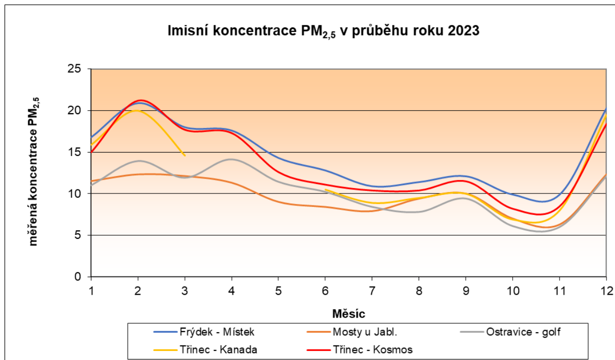
Obrázek 29 Roční chod imisních koncentrací PM 2,5 v roce 2023 [μg/m 3 ] Okres Frýdek-Místek
